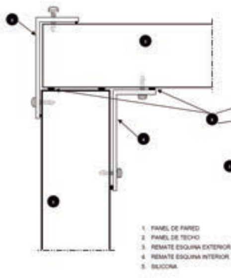
ENTREGA PANEL CONGELACIÓN
