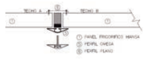
SUSPENSIÓN TECHO POR OMEGA
