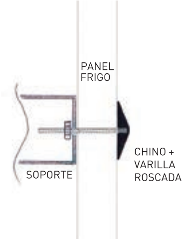
SOPORTE FACHADA POR CHINO
